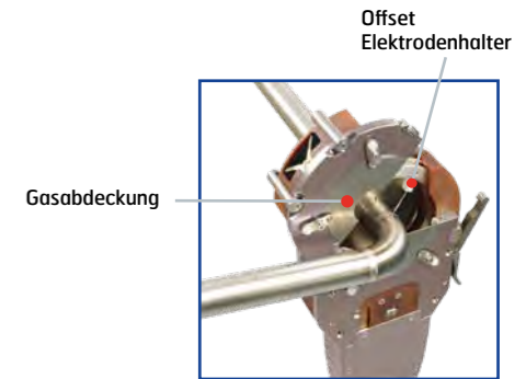
Rohrbogen-Kit
